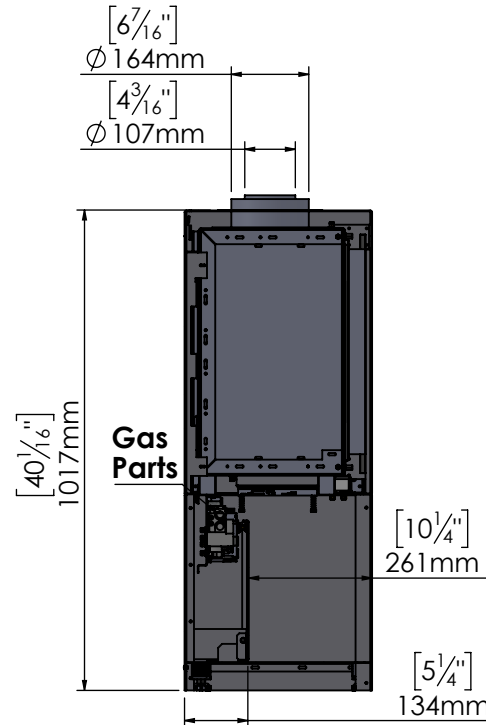
SECTION A-A SCALE 1 : 16
