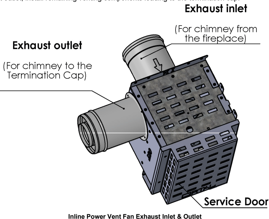
Inline Power Vent Fan Exhaust Inlet & Outlet
